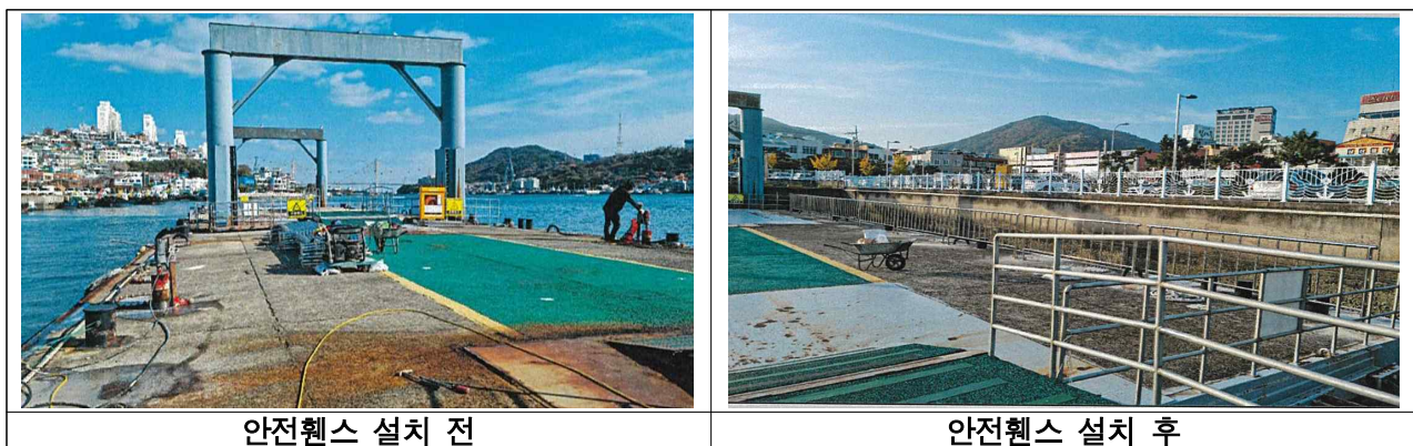
[사진 3] 여수연안여객선터미널 부잔교 내 안전휀스 설치현황
